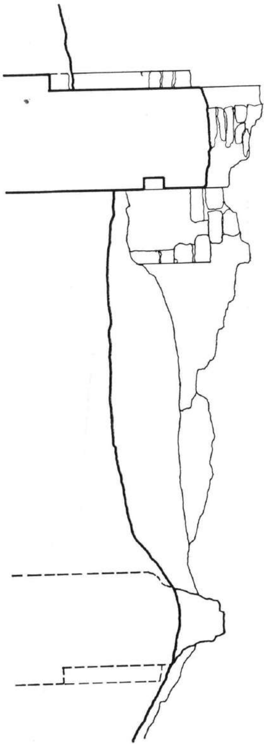
Ст. 8 Русевине цркве на Руднику, подужни пресек (цртеж арх. С. Ђорђевића)
