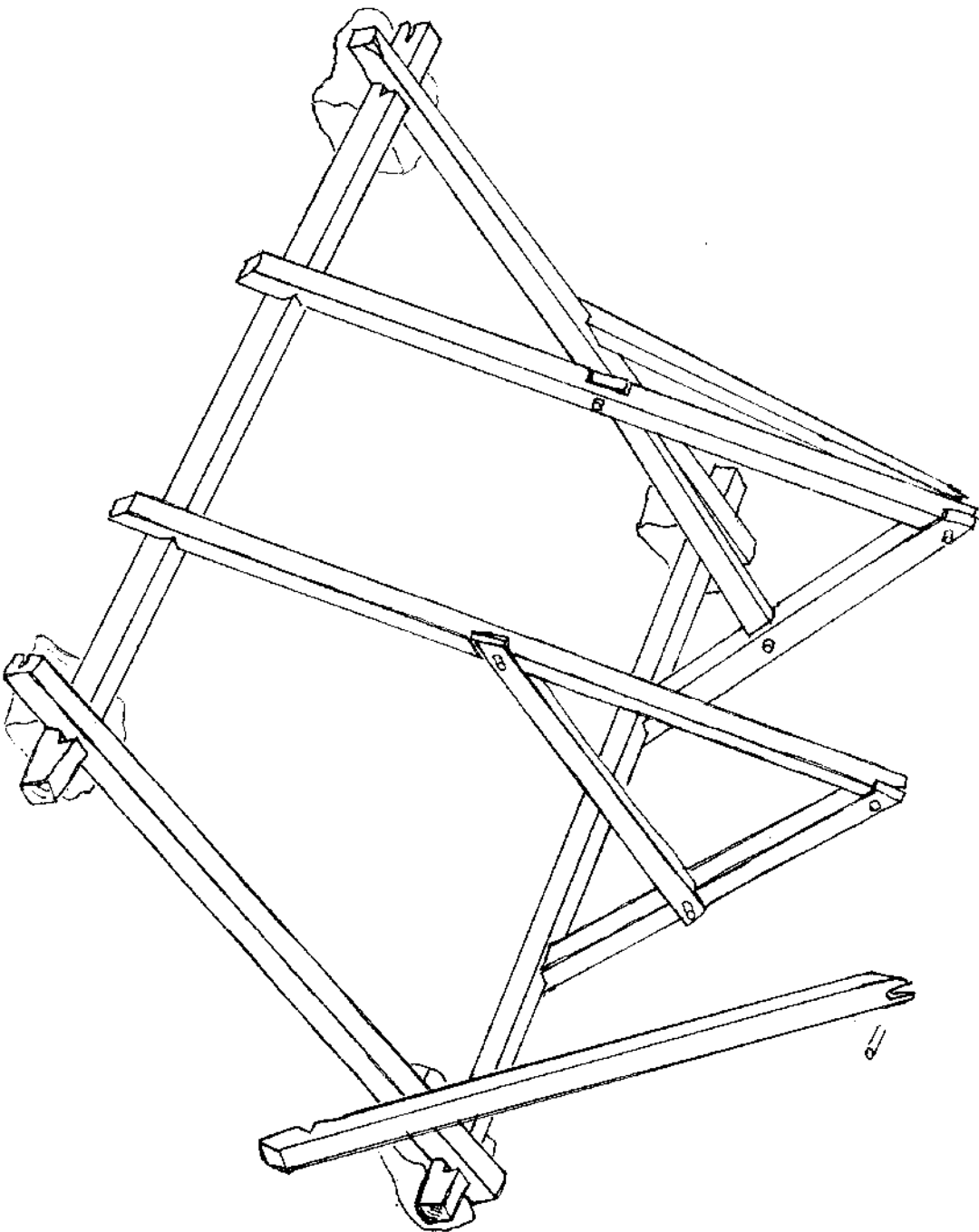
Прек 2 Стајање полова са гредом „Думењакром“ Dessins 2 jointure des poutres latérales et de la poutre frontale
