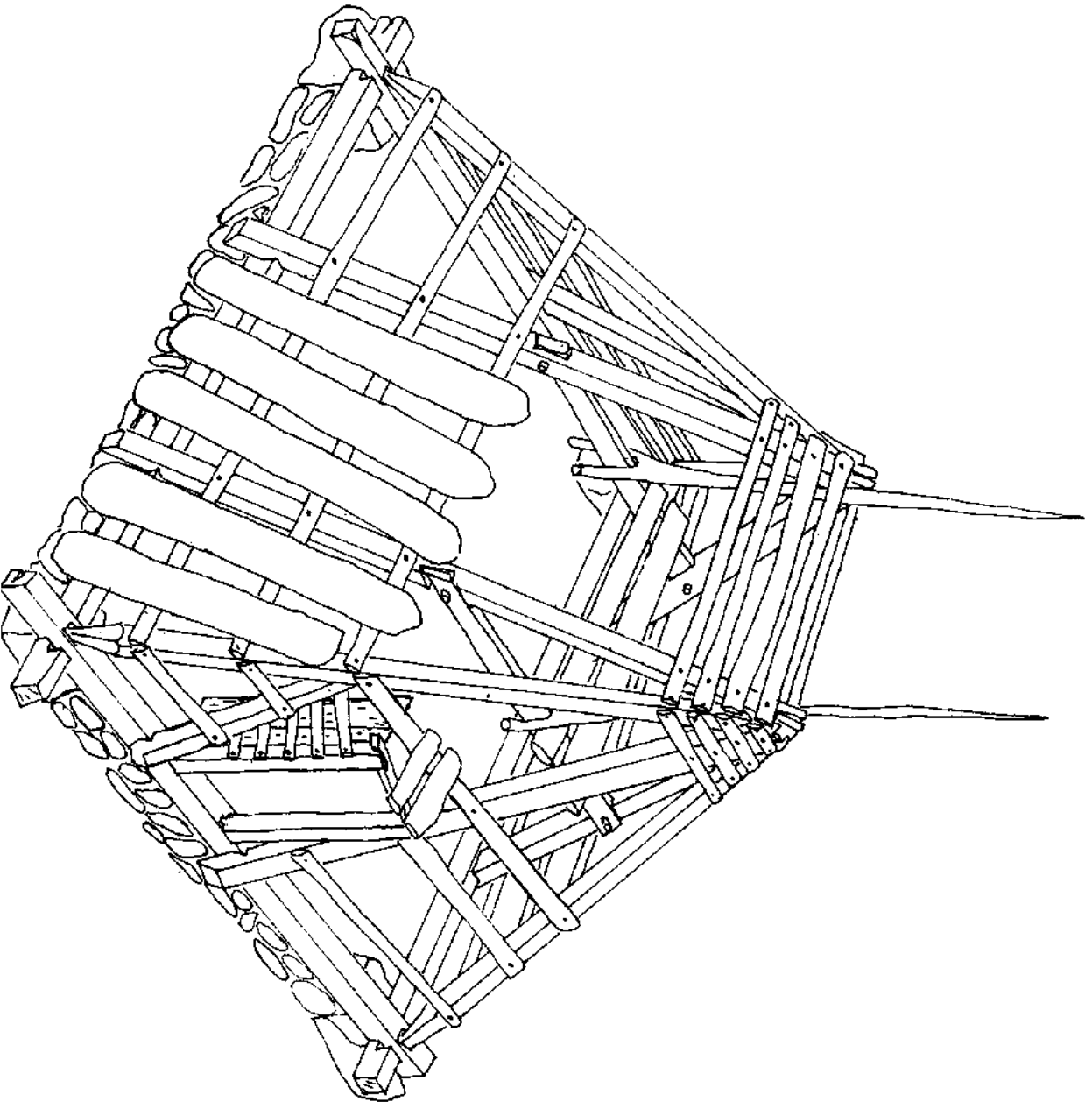
Цртеж 4 Дрвена конструкција сибаре Dessins 4 Charpente de bois de la cabane de bergers
