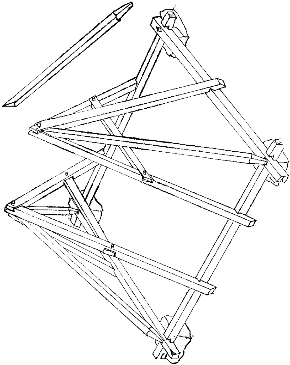
Цртеж 3 Снајажне греде „маије“ са „главом пога“ Dessins 3 Jointure de la poutre angulaire et du faite
