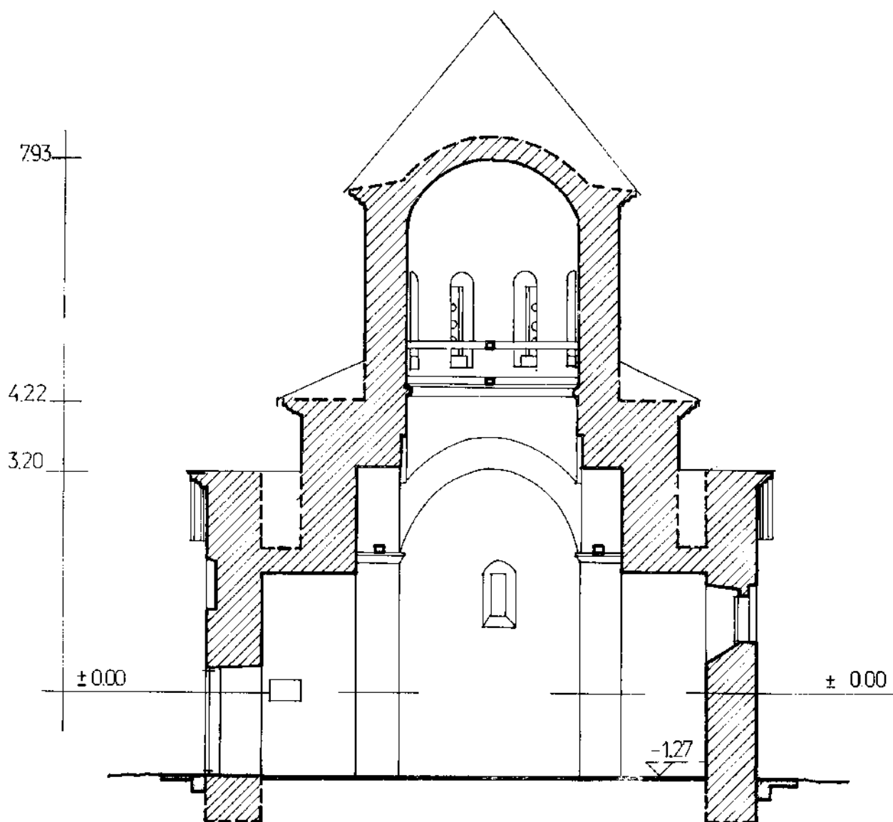
Сл. 3 Пресек б-б Сорре b-b
