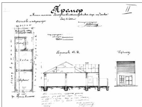
Сл. 2. – План дућана Влајка Антонијевића трговца из Чачка у Улици Краља Милана, збирка породице Ђирковић
