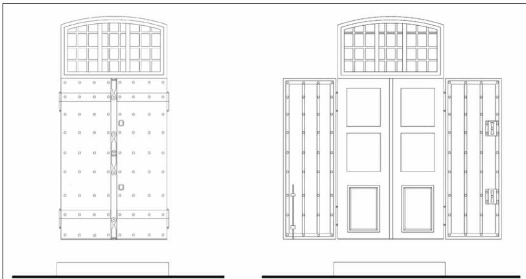
Сл. 17. – Детаљ улазних врата са капцима кројачке радње Бугарчића у Улици Драгише Мишовића у Чачку, технички снимак аутора
