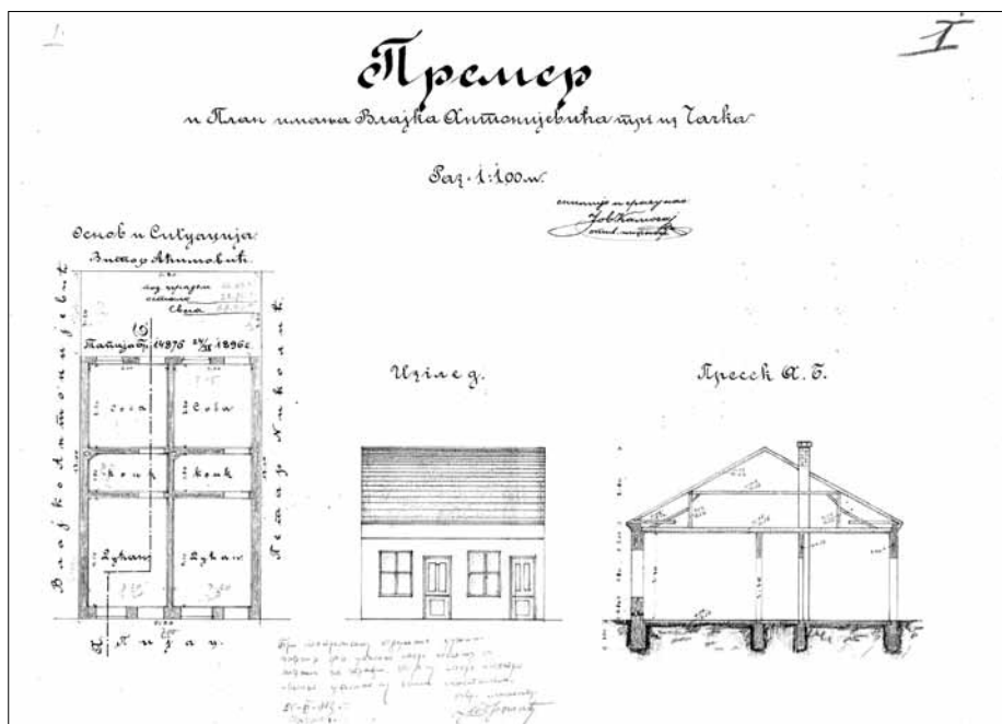
Сл. 4. – План двојног дућана Влајка Антонијевића у Чачку, збирка породице Ђирковић
