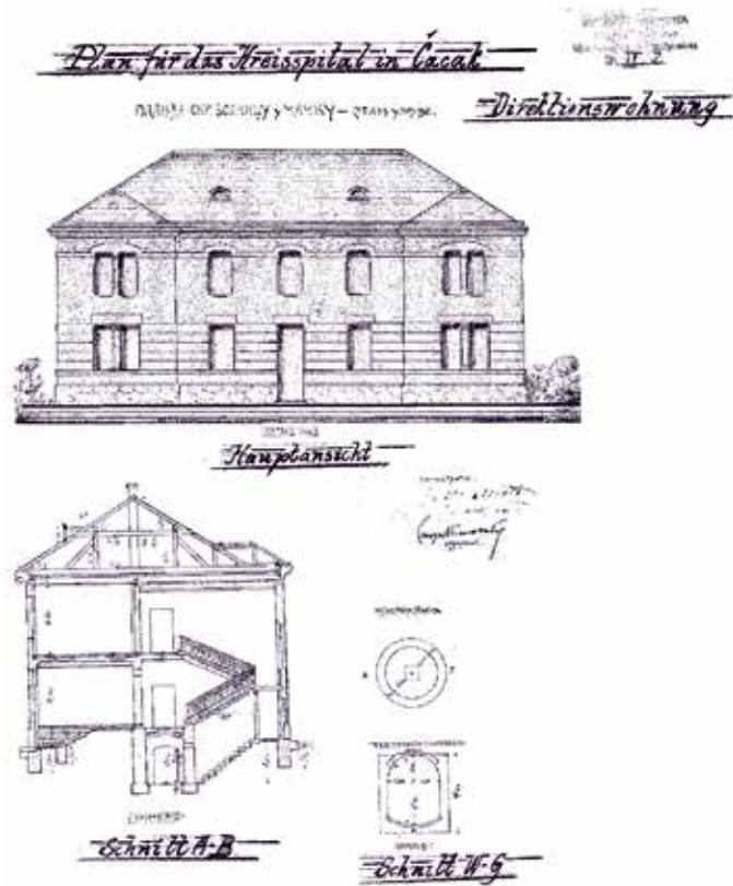
Сл. 10: Збирка Архива Министарства грађевина у Београду: план уйравне зїраде болнице
