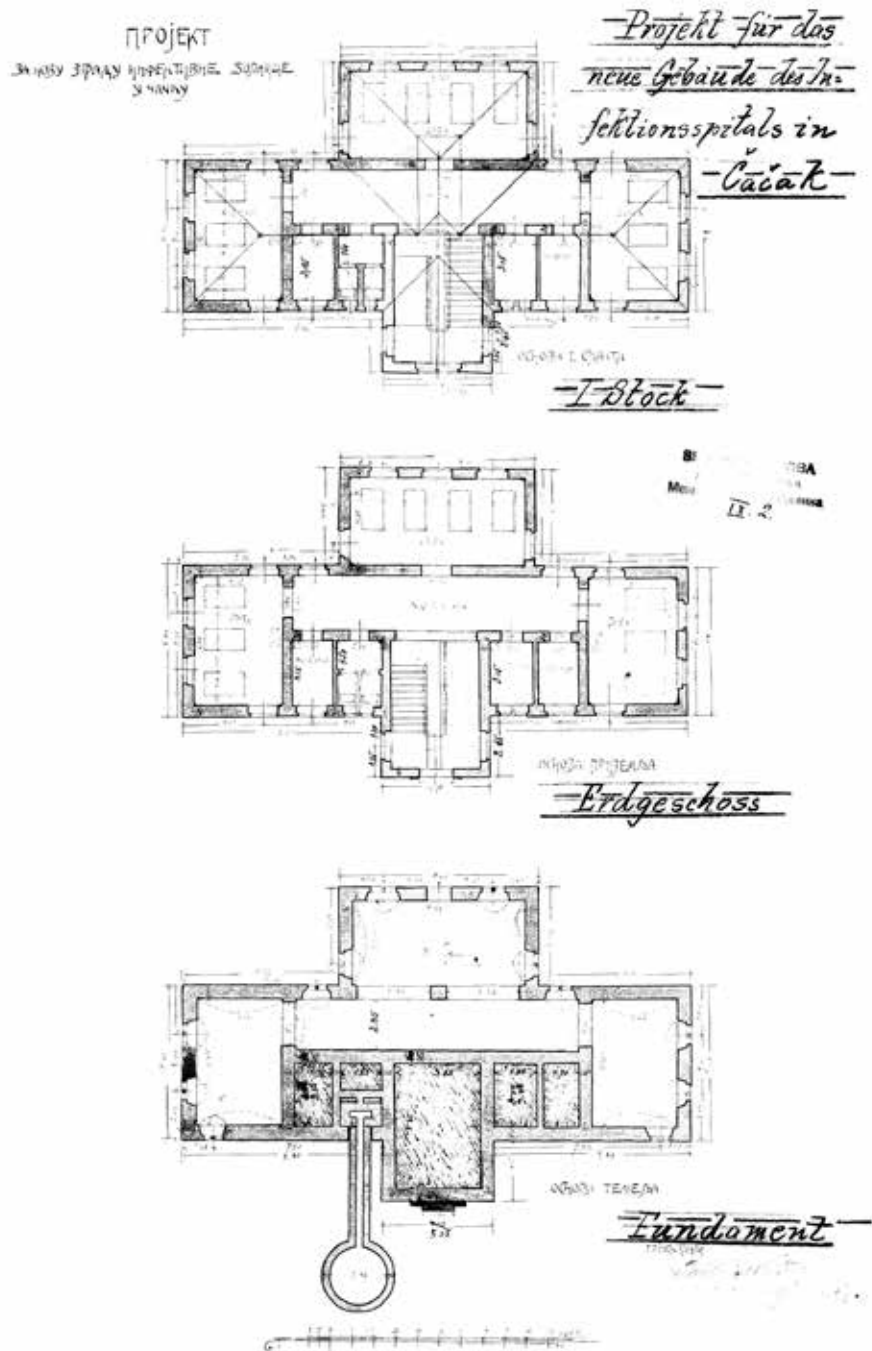
Сл. 9: Збирка Архива Министарства грађевина у Београду: план Инфективне болнице у Чачку
